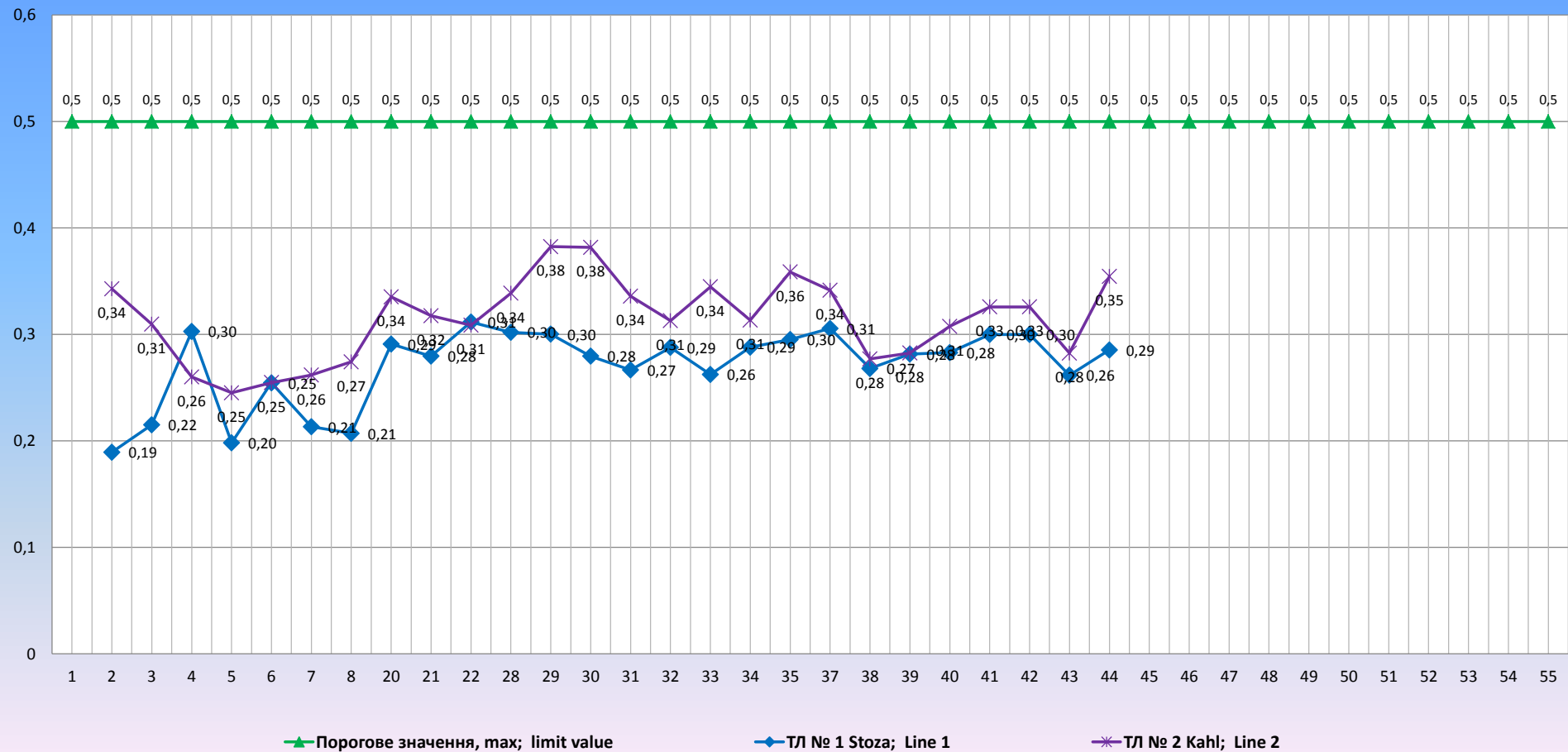
Середні фактичні показники вмісту пилу (< 3,15 мм) в ДПГ в 2021 році The average fines (< 3,15 mm) of the pellets in 2021
